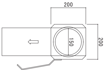
{ フィルターユニット平面図 }
